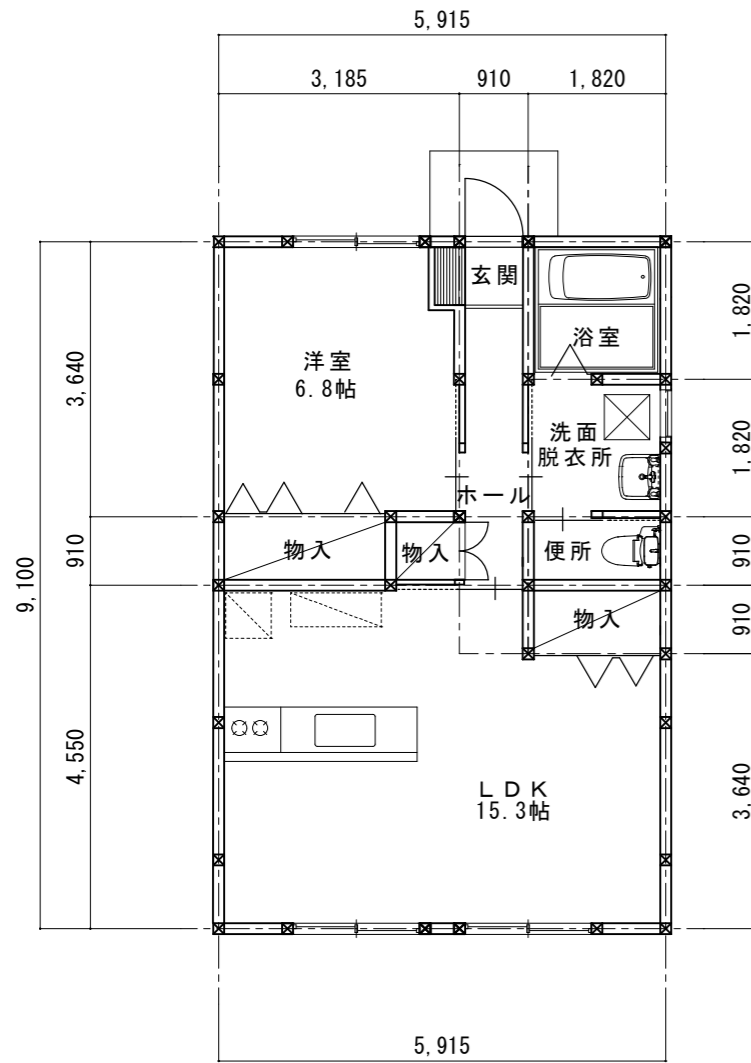
1LDK 53.8㎡
