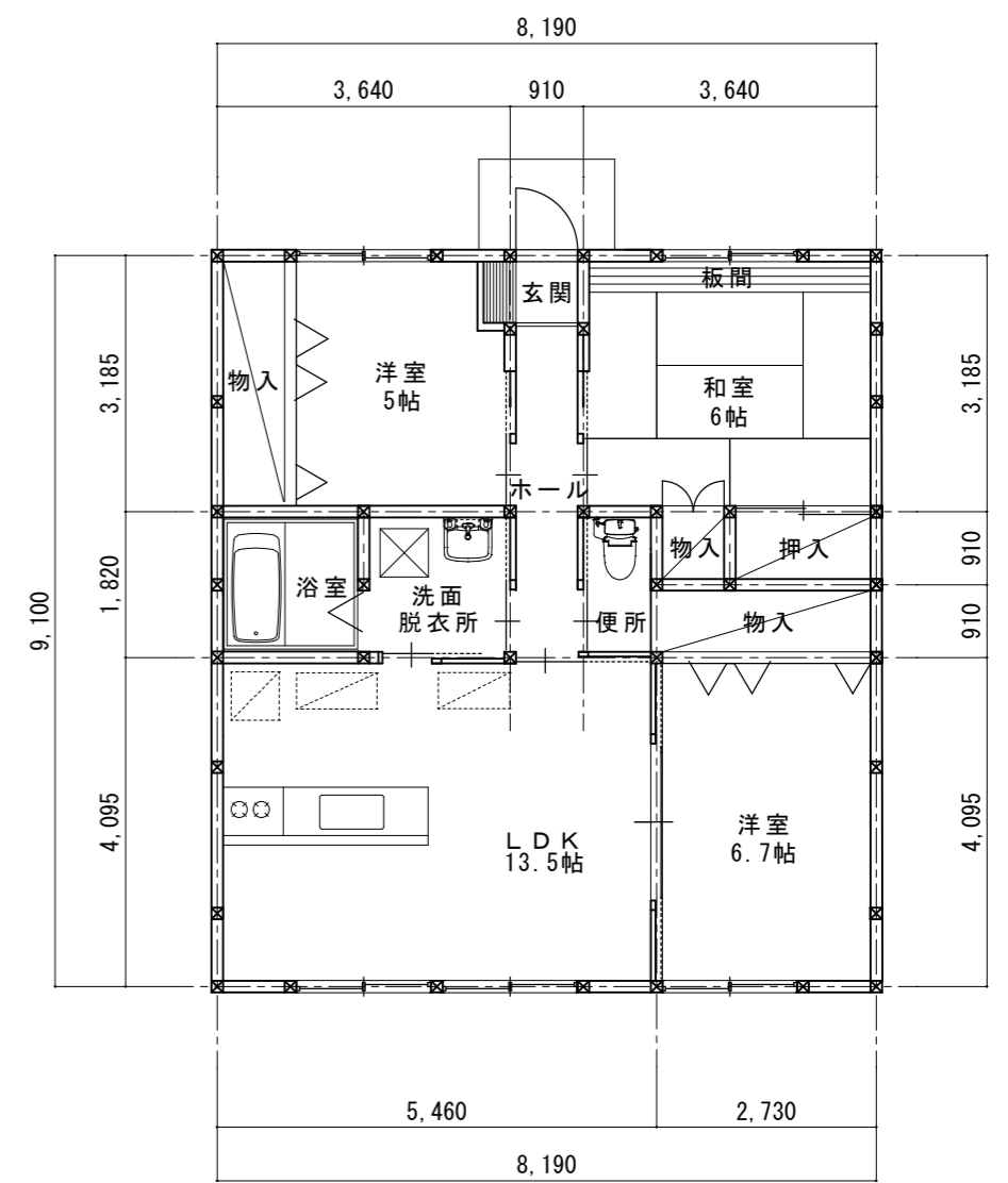
3LDK 74.5㎡
